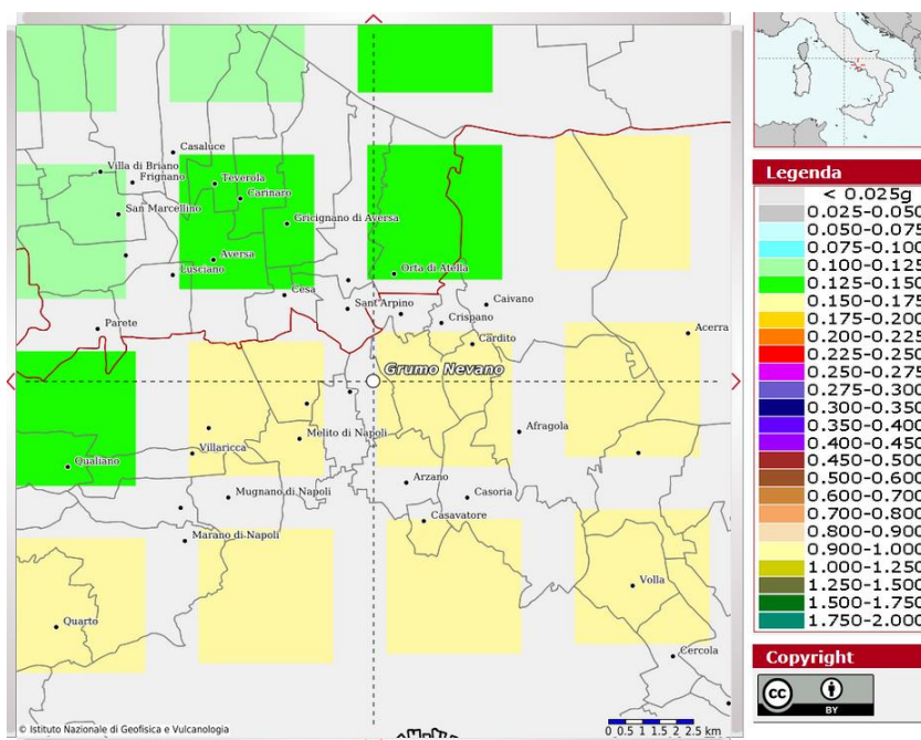
Mappa della pericolosità sismica del territorio comunale di Grumo Nevano (NA) dell'INGV con i range di valori delle ag nella legenda corrispondente
